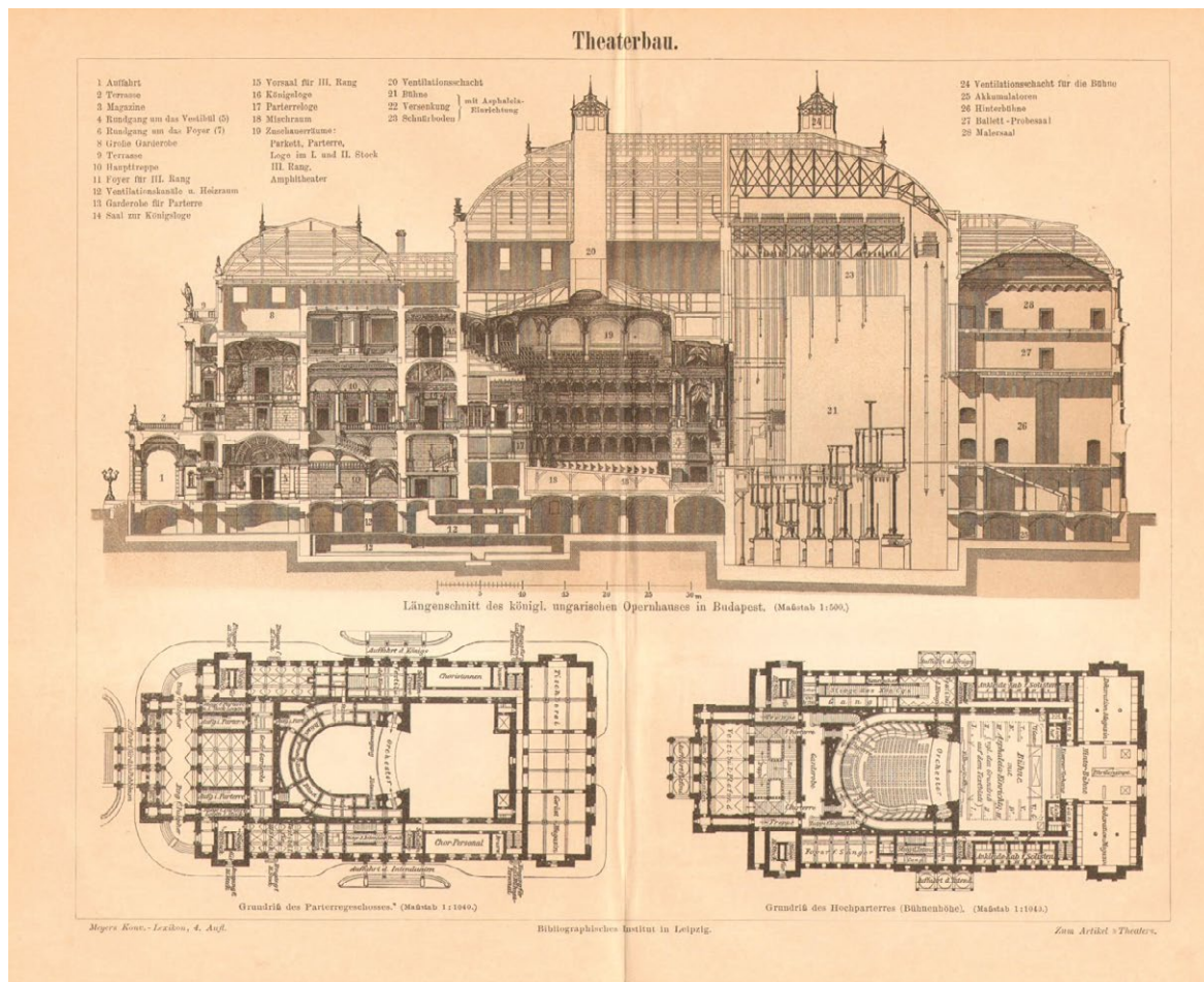
Az Operaház hosszmetsete és alaprajzai, Meyers Konversationslexikon, 1885
